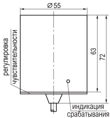
Габаритный чертёж
